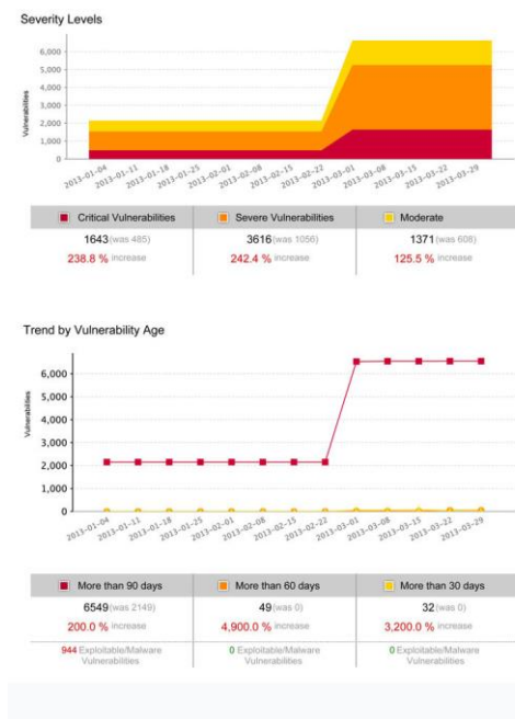
Grafik: Zeitliche Entwicklung von gefundenen Schwachstellen
